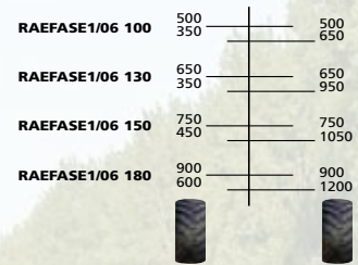
SPOSTAMENTO - OFFSET
